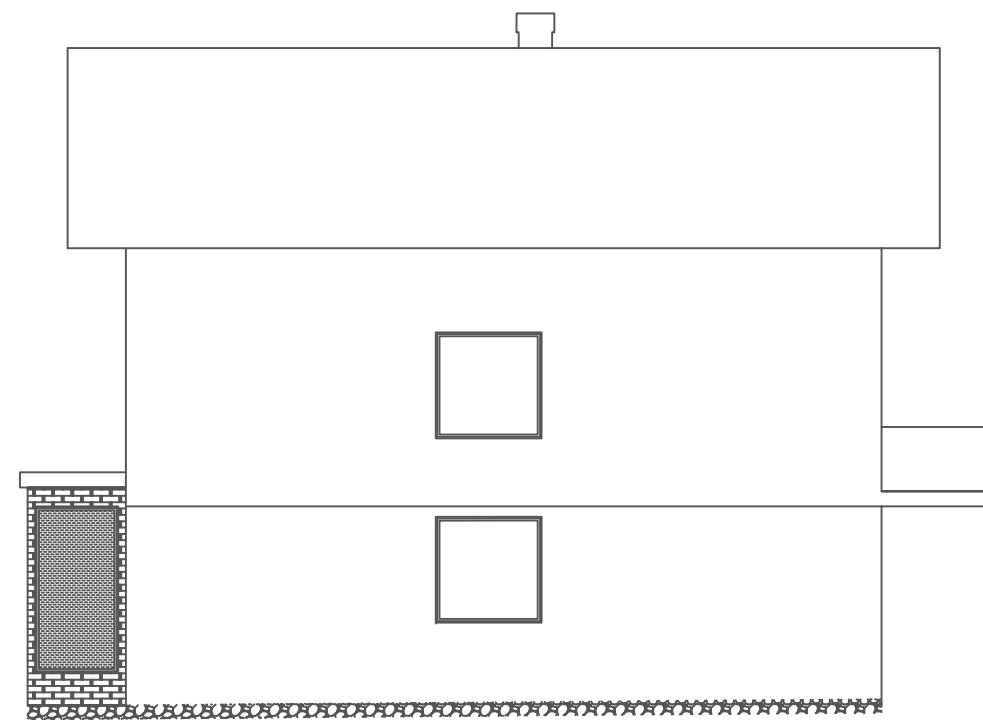
СЕВЕРНА ФАСАДА
