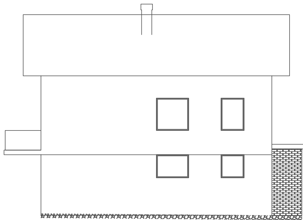
ЈУЖНА ФАСАДА
